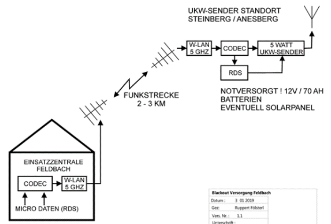
Abbildung 3: Skizze Bestandteile eines Notradiosenders
